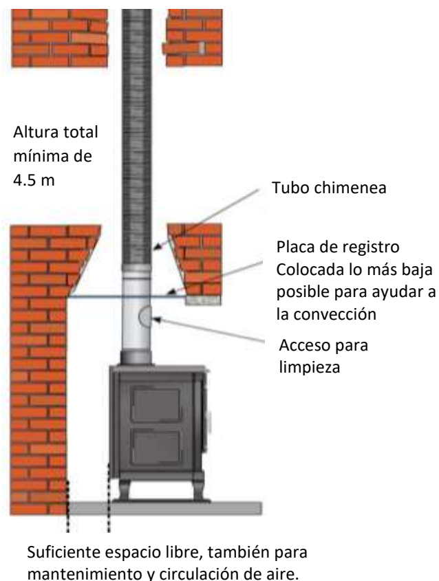
Fig. 3.- Ejemplo de conexión a una chimenea de obra
