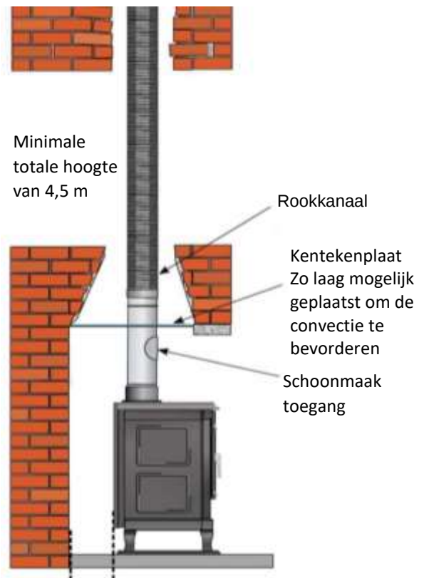
Afb. 3.- Aansluitingsvoorbeeld aan een gemetselde schoorsteen
